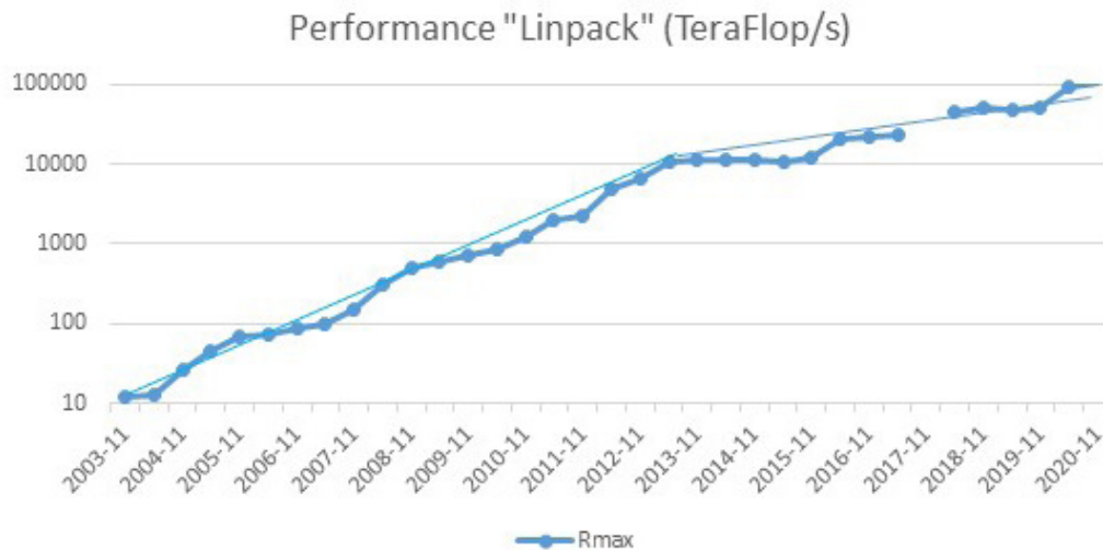
Figure 1 : Évolution de la puissance moyenne des dix superordinateurs les plus puissants
