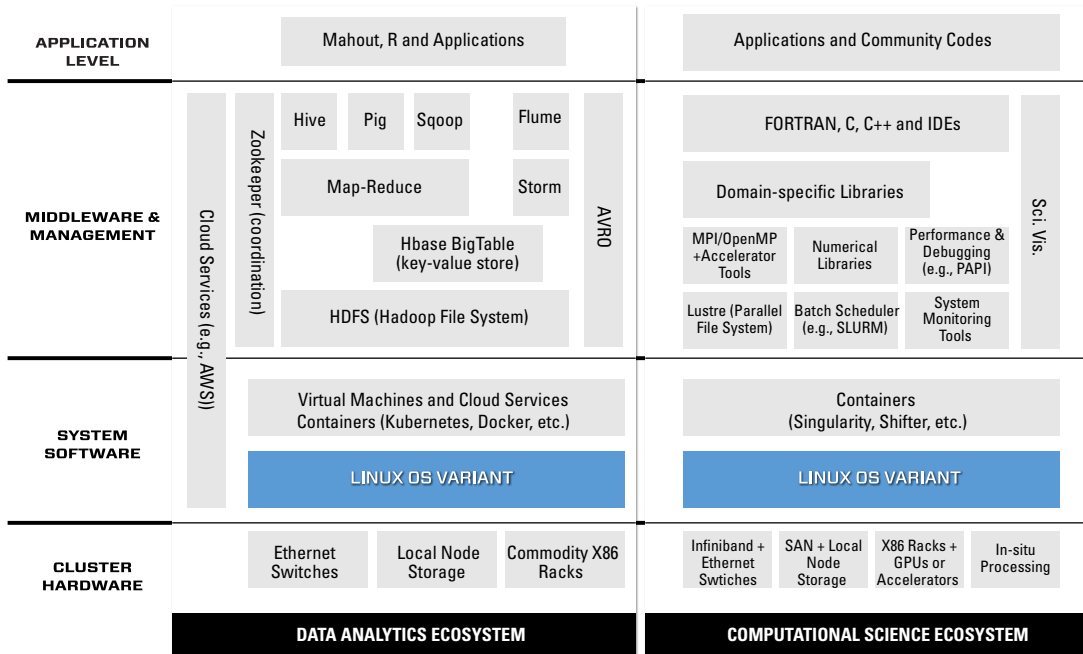
Figure 3 : Les différents types de logiciels utilisés pour le traitement des données massives (HPDA, à gauche) et le calcul scientifique (HPC, à droite). Source : Asch et al. , 2018.
