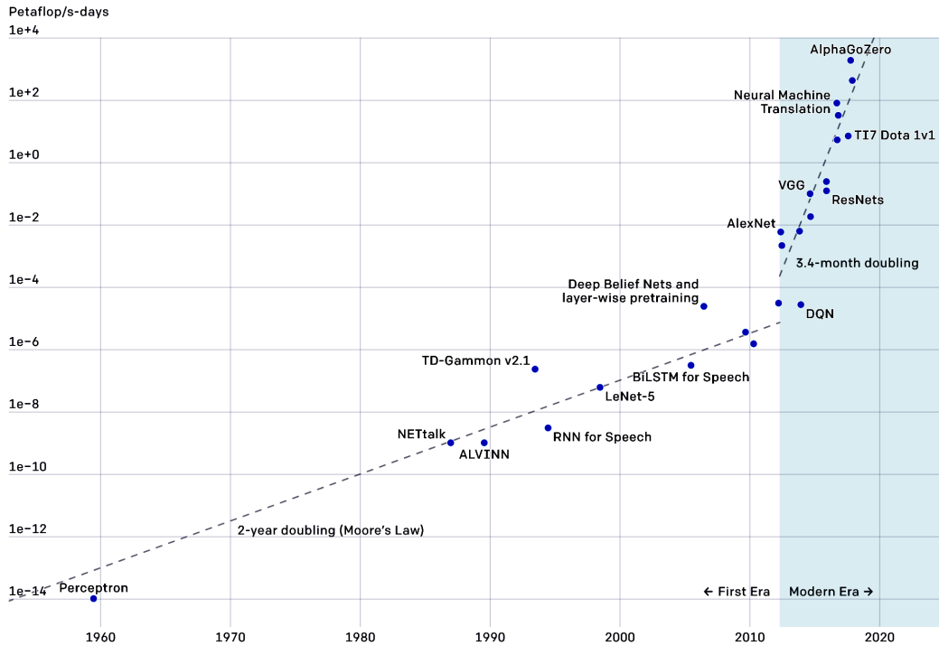
Figure 4 : L'explosion des besoins en puissance de calcul pour l'apprentissage de modèles (vision, traitement de langages et jeux). Source https://openai.com/blog/ai-and-compute
