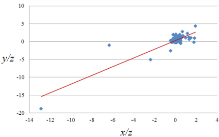
Corrélation entre les quotients x/z et y/z
