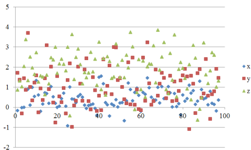
Tirages des trois variables x,y et z
